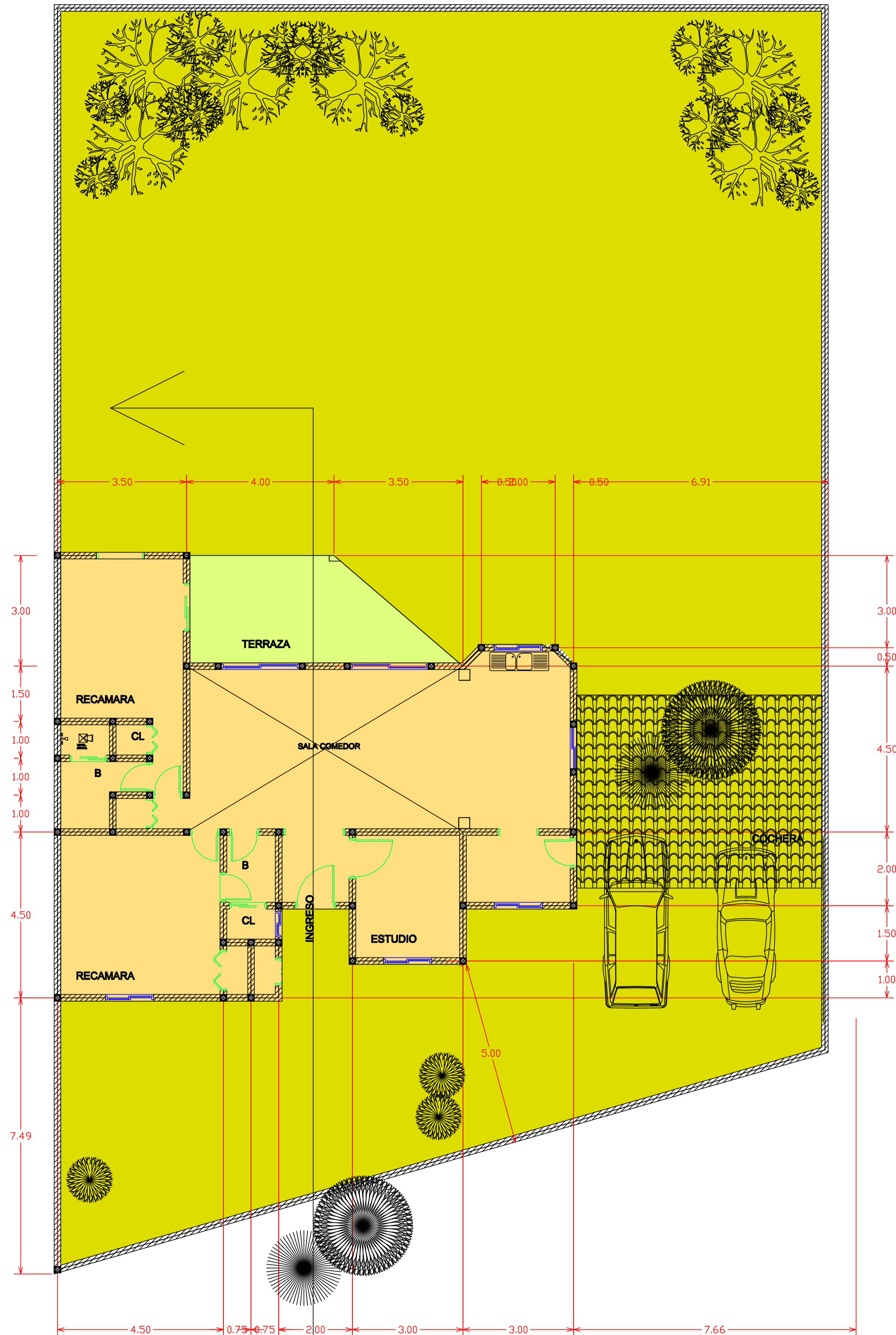
PLANTA ARQUITECTONICA
